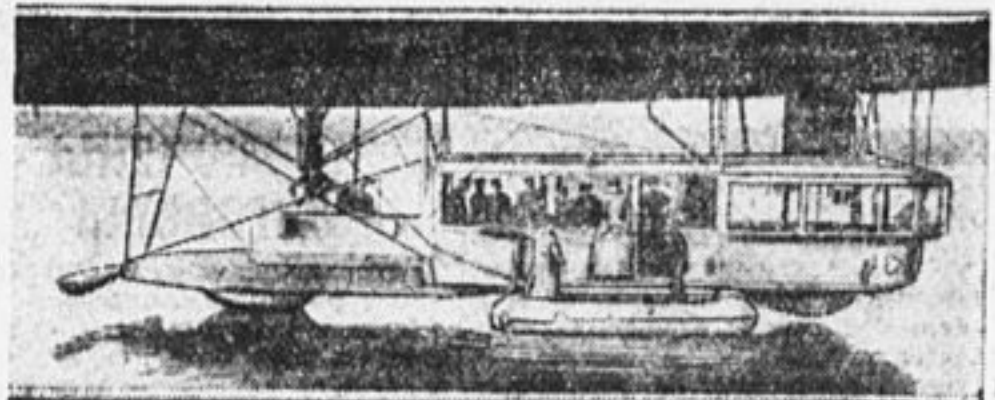
Приспособление под гондолой «Цепелина» для опускания на воду.
